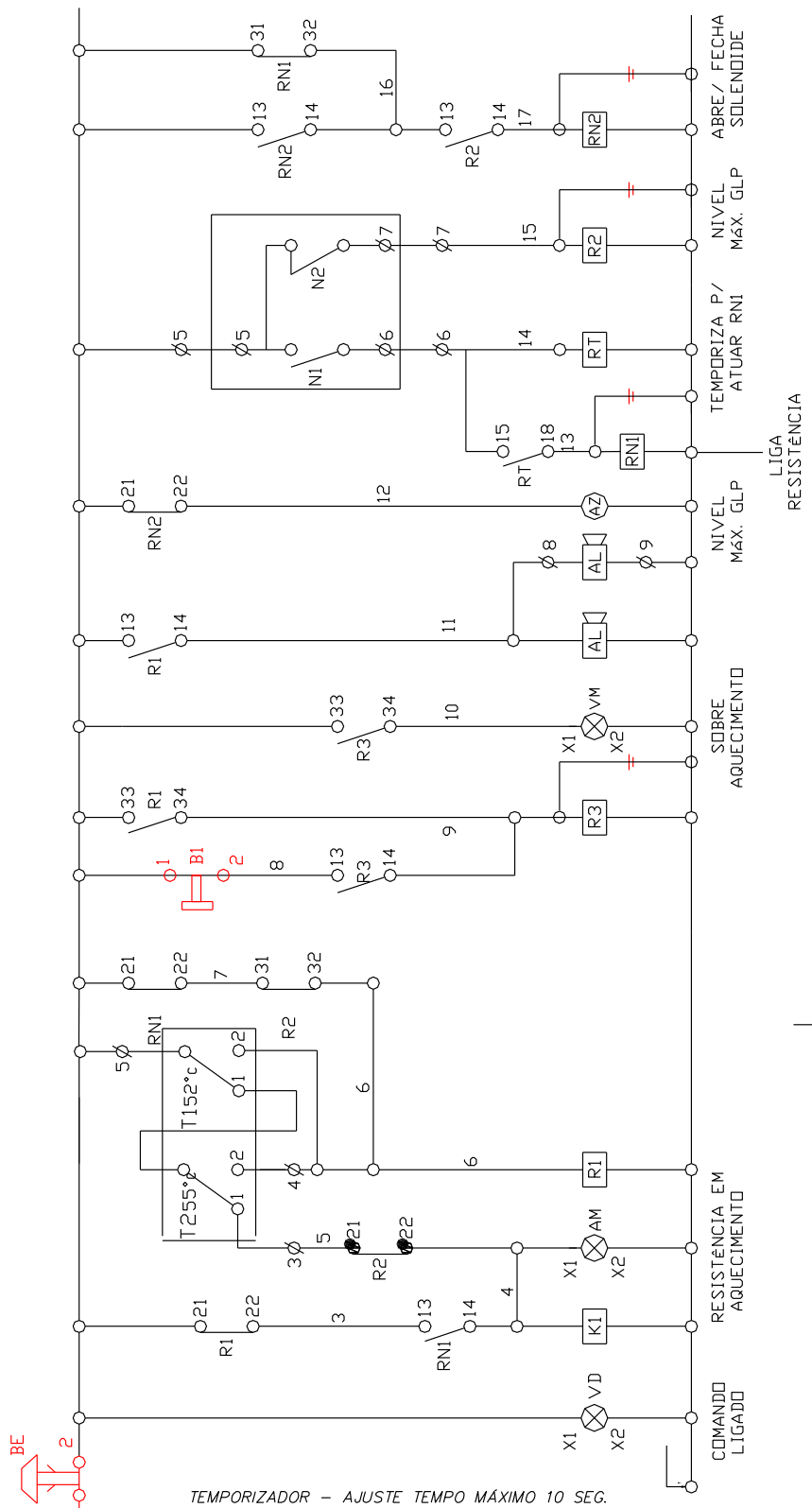
TEMPORIZADOR - AJUSTE TEMPO MÁXIMO 10 SEG.
